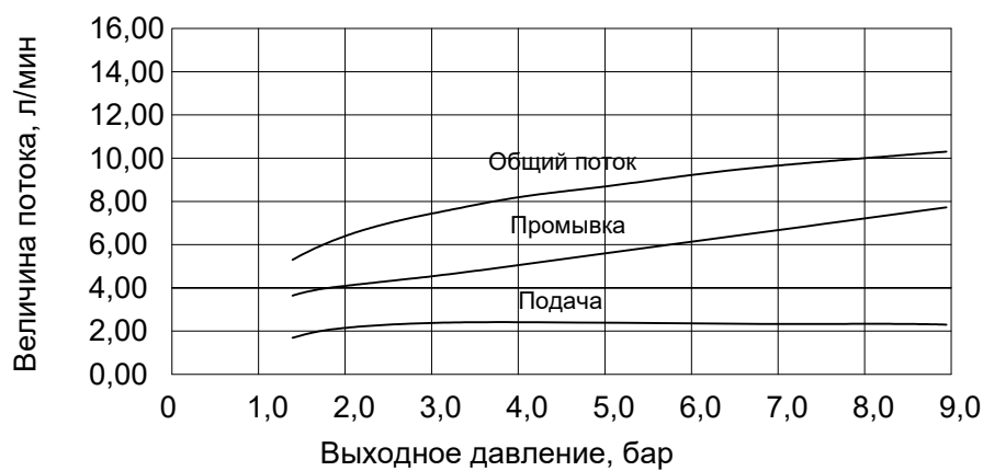
Инжектор 4
