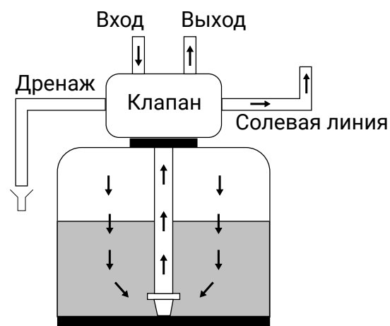
Заполнение бака-солеорастворителя
