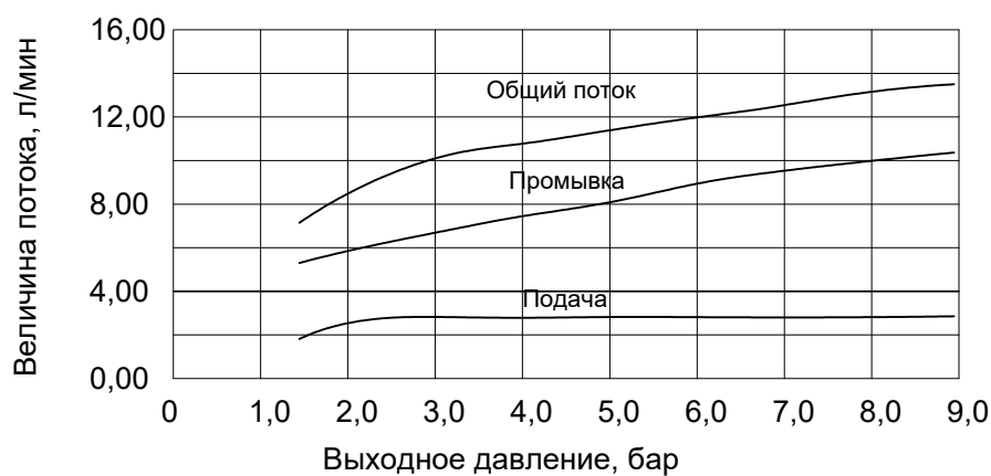
Инжектор 5
