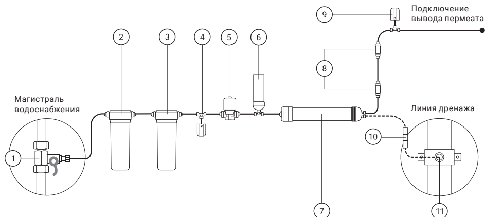
Рис. 1. Схема подключения Гейзер Лайн 1500/4000.
