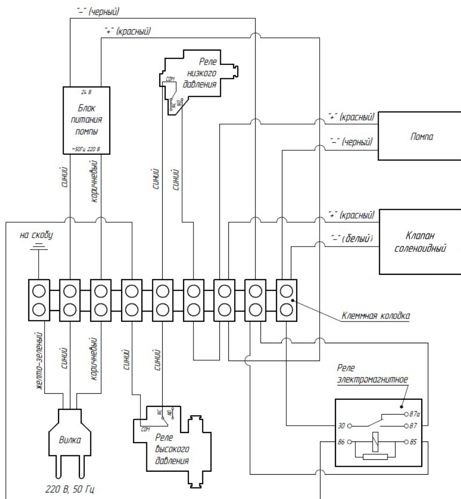
Рис. 14. Схема для Гейзер Лайн 1500.
