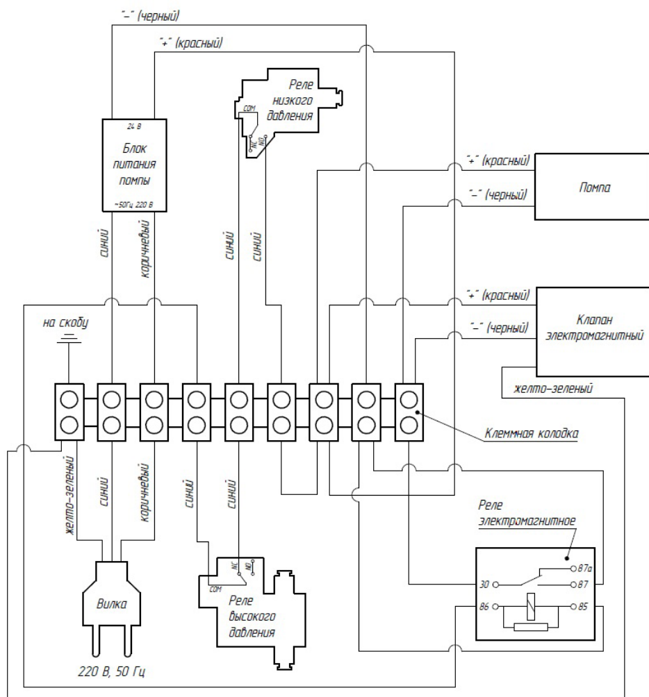
Рис. 15. Схема для Гейзер Лайн 4000.
